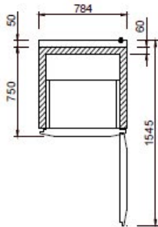
ABBATTITORE A TEGLIE AVANT 5T +90°C -18°C al cuore
