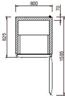
ABBATTITORE A TEGLIE AVANT 5T +90°C -18°C al cuore
