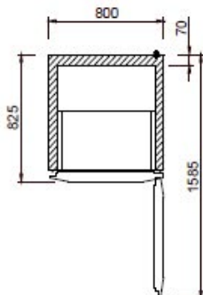
ABBATTITORE A TEGLIE AVANT 15T +90°C -18°C al cuore
