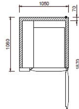
ABBATTITORE A TEGLIE AVANT 15T +90°C -18°C al cuore
